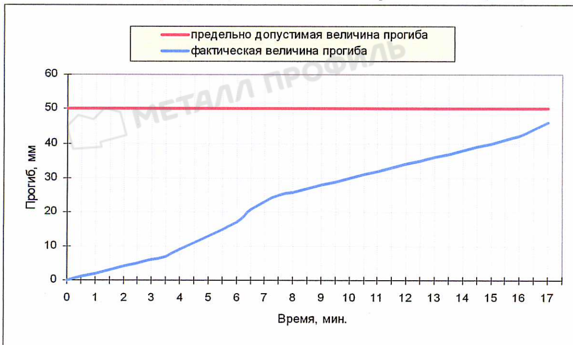
Рис. 3. График изменения величины прогиба конструкции.
