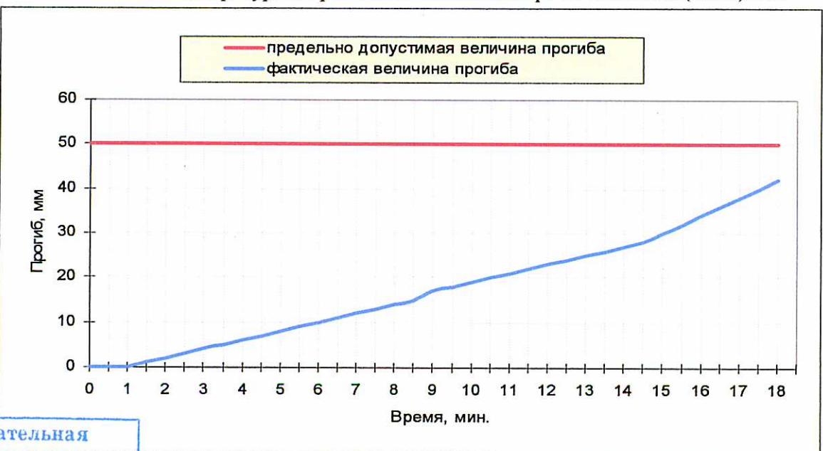
Рис. 9. График изменения величины прогиба конструкции.
