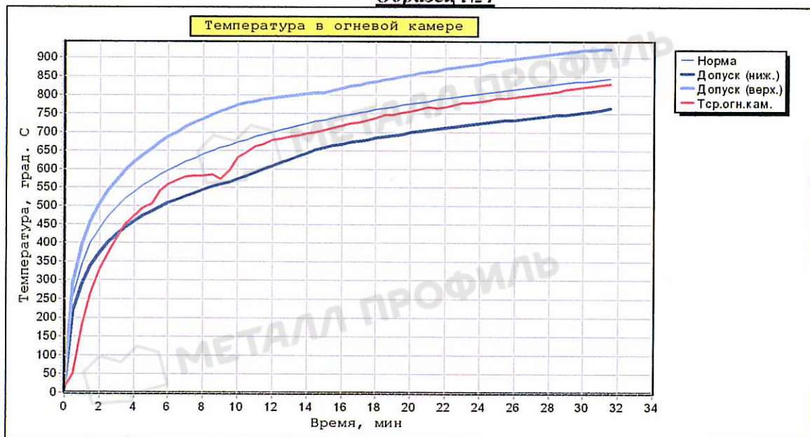
Рис. 11. Температурный режим в огневой камере «Установки (печи)...».
