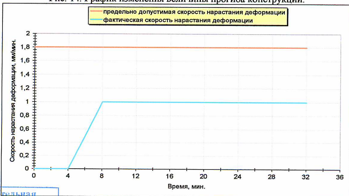
Рис. 15. График изменения скорости нарастания деформации конструкции.
