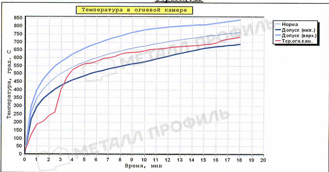
Рис. 8. Температурный режим в огневой камере «Установки (печи)...
