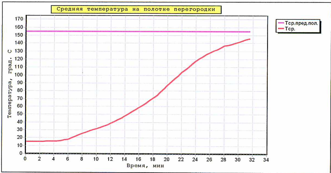
Рис. 13. График среднего значения температуры на необогреваемой поверхности перегородки.
