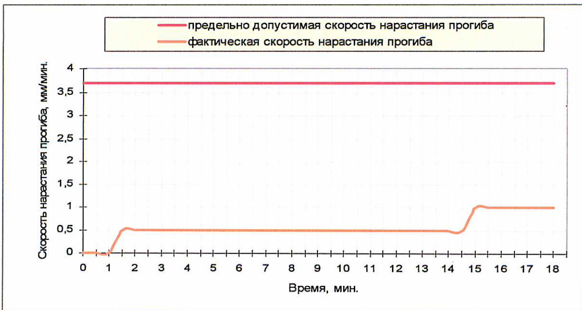
Рис. 10. График изменения скорости нарастания деформации конструкции. Образец №4
