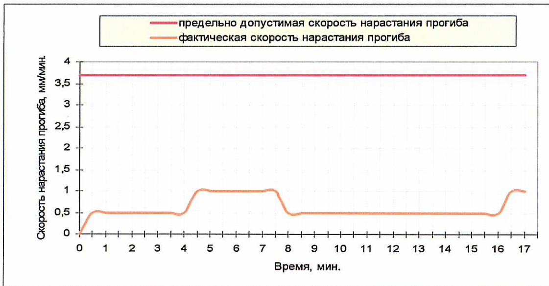
Рис. 4. График изменения скорости нарастания деформации конструкции.
